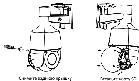
Снимите заднюю крышку
